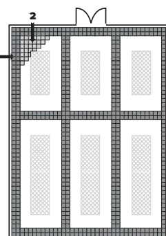
Obr. č. 6 Instalace kolem fixních předmětů - postup kladení dlaždic
