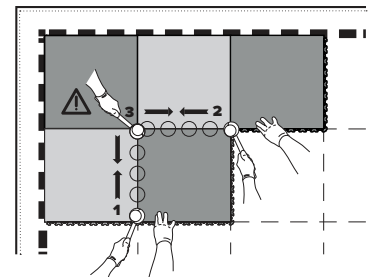
Obr. č. 4 Způsob pokládky dlaždic INVISIBLE, BUSINESS
