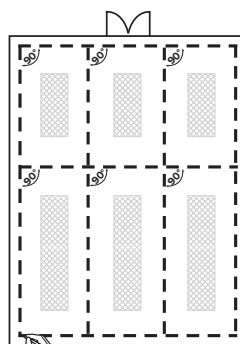
Obr. č. 5 Instalace kolem fixních předmětů - vytčení linií
